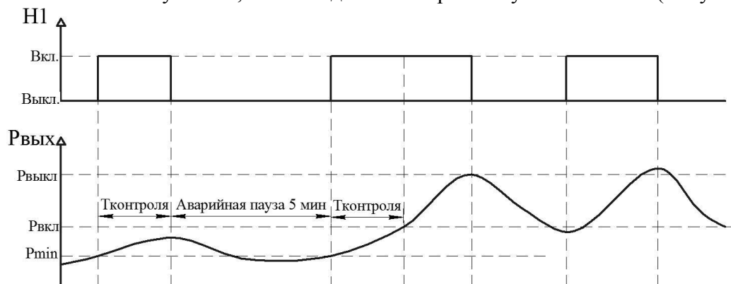
Рисунок 21 – Диаграмма работы БУН в режиме «ПОДДЕРЖКА Р»
