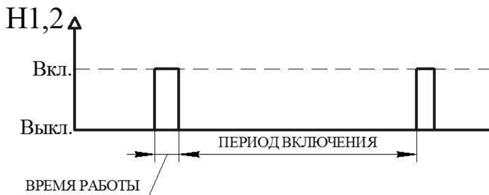
Рисунок 19 – Диаграмма работы БУН в режиме «МЕЖСЕЗОН»
