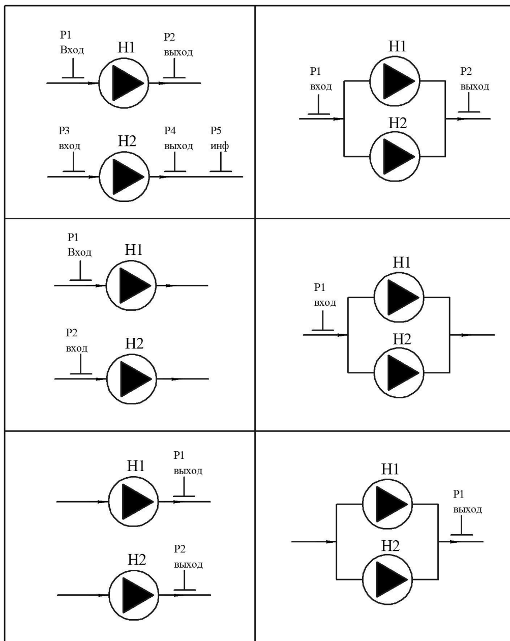
Рисунок 24– Расположение и назначение датчиков давления относительно насосов
