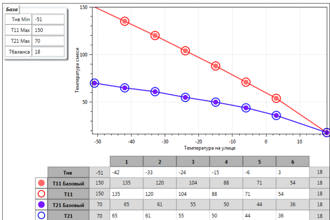
Рисунок 45 – Узловые точки графиков теплоснабжения
