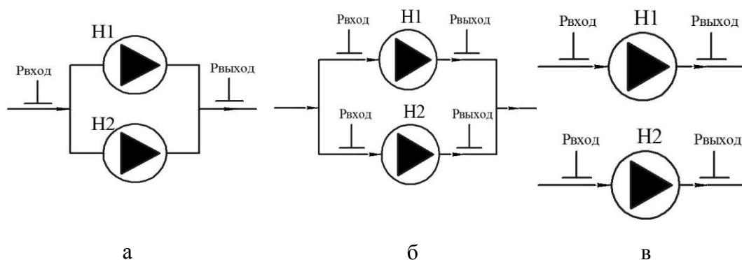
Рисунок 17– Схема а - двояного насоса, б – насосной группы, в – независимые насосы (раздельная схема управления)
