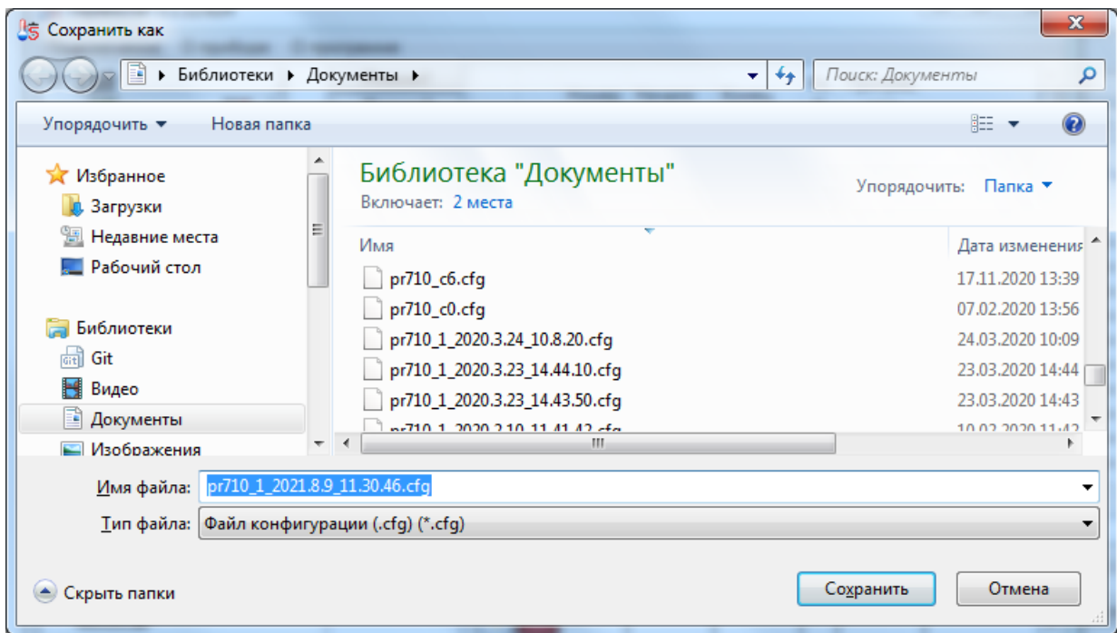
Рисунок 67 – Окно сохранения
