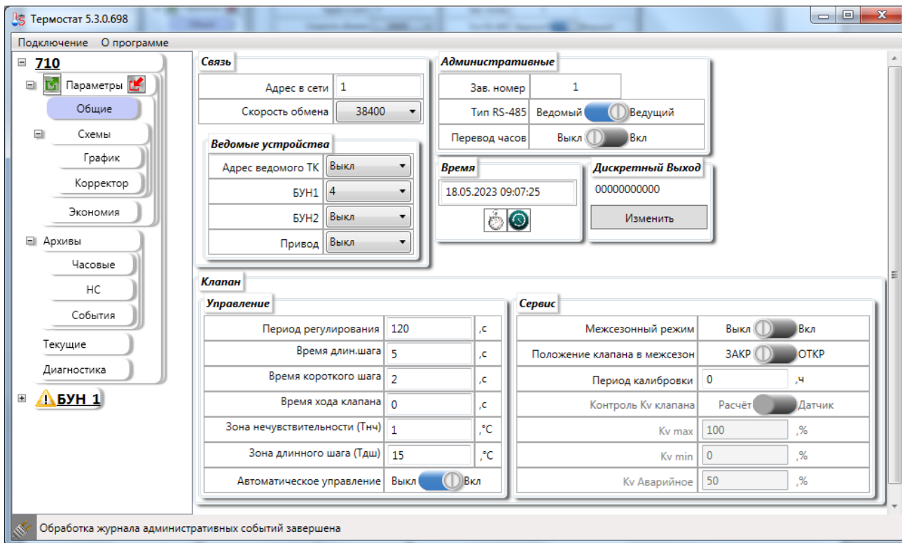
Рисунок 33 –Вкладка «Общие»
