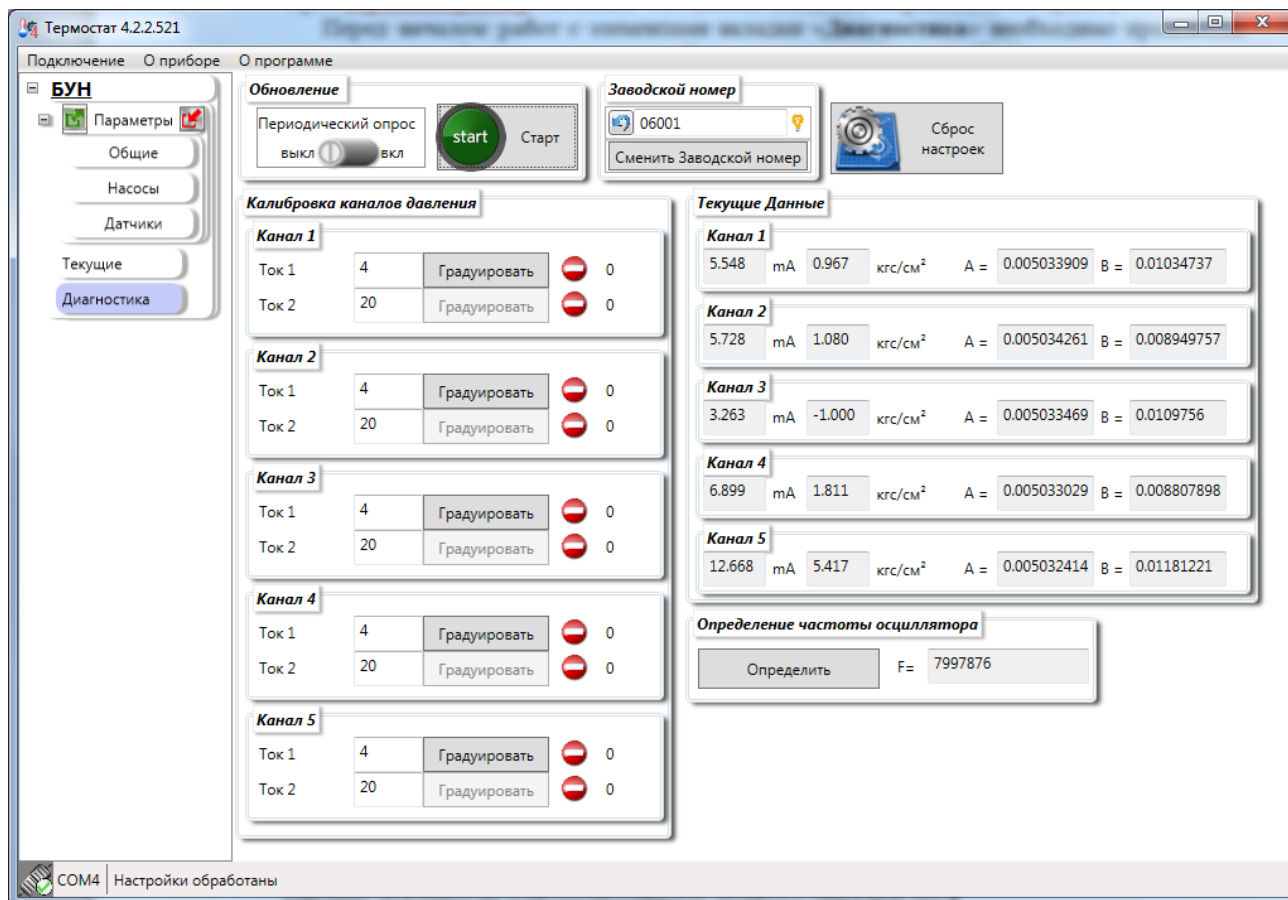
Рисунок 29 – Вкладка «Диагностика»
