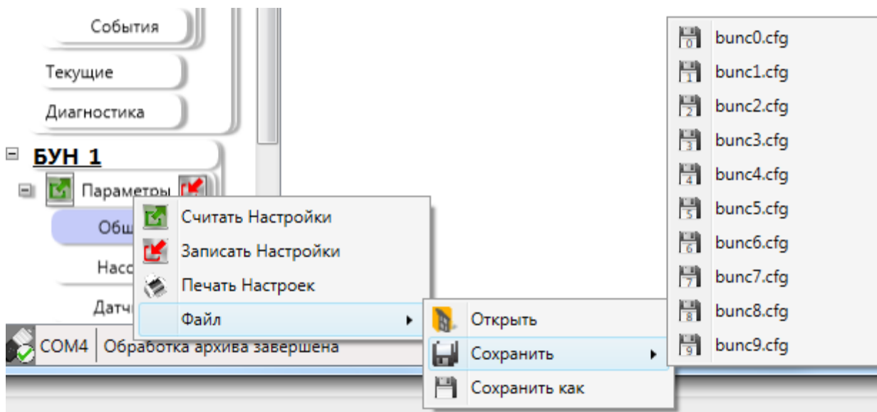
Рисунок 99 – Меню «Сохранить»
