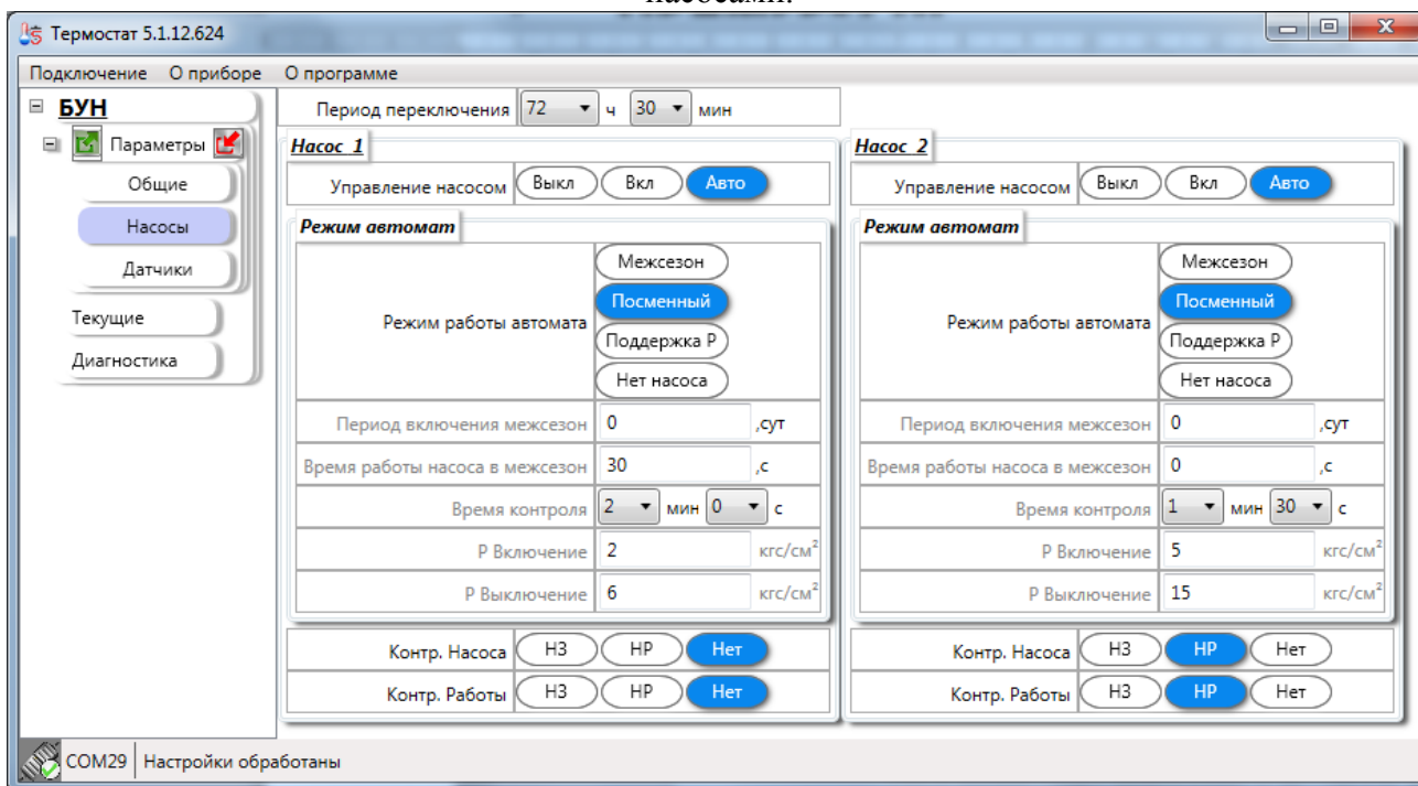
Рисунок 18 – Параметры насосов
