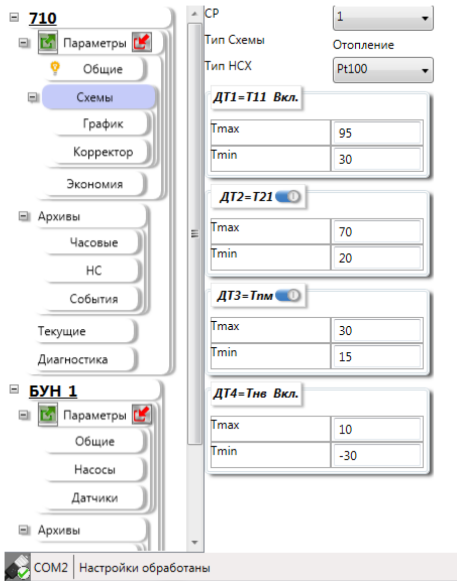
Рисунок 43 – Вкладка «Схемы»
