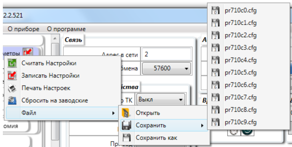
Рисунок 63 – Меню «Сохранить»
