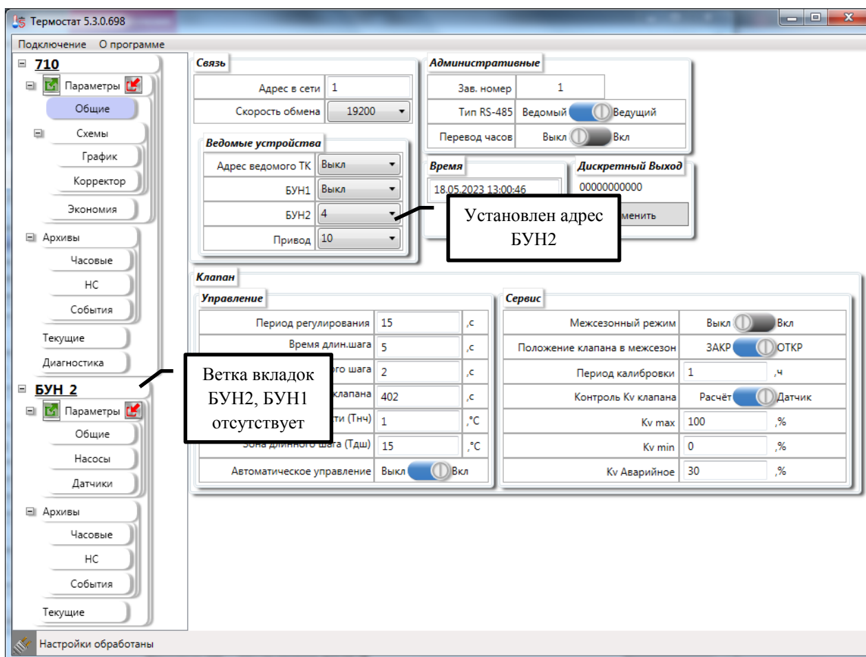
Рисунок 95 – Подключен БУН2
