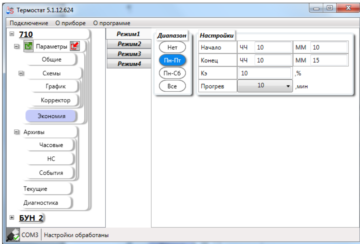
Рисунок 50 – Вкладка «Экономия»
