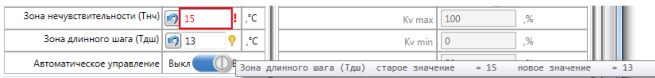
Рисунок 41 – Обработка ограничений
