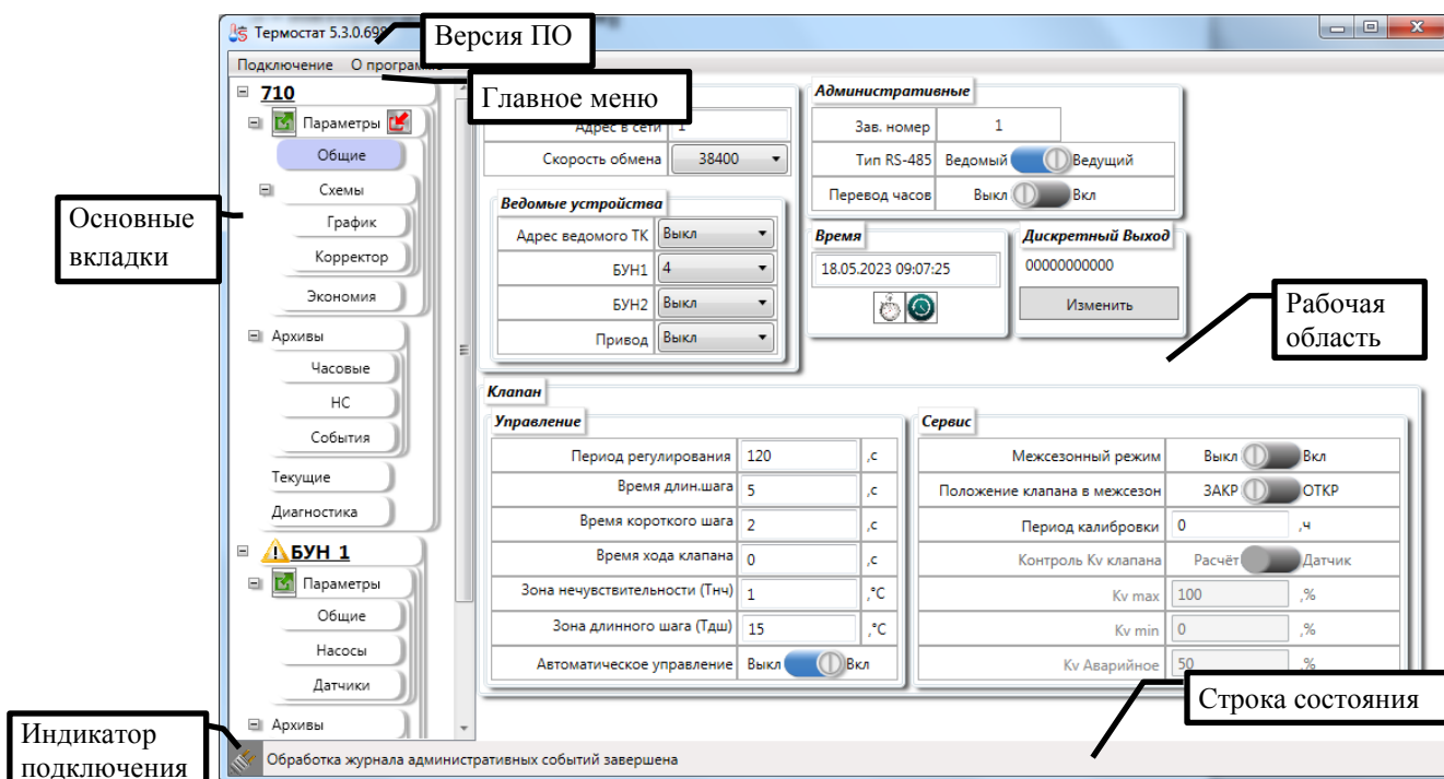
Рисунок 4 - Стартовый экран
