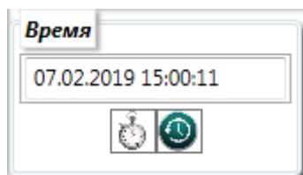
Рисунок 36 – настройки времени
