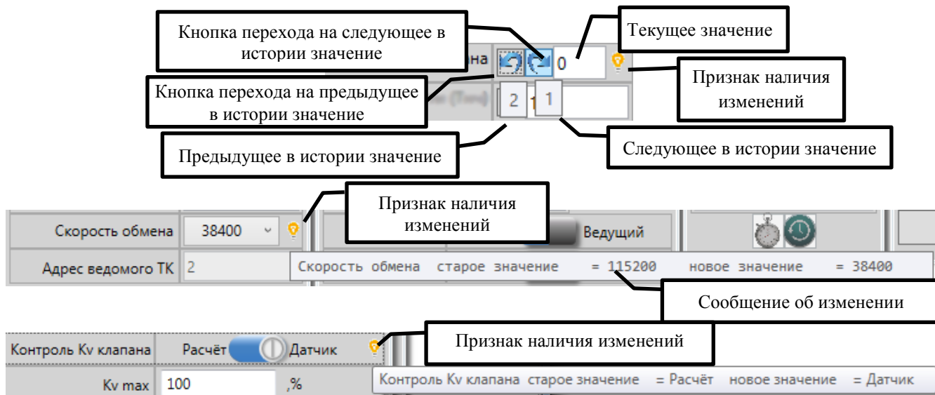
Рисунок 12 – Представление полей
