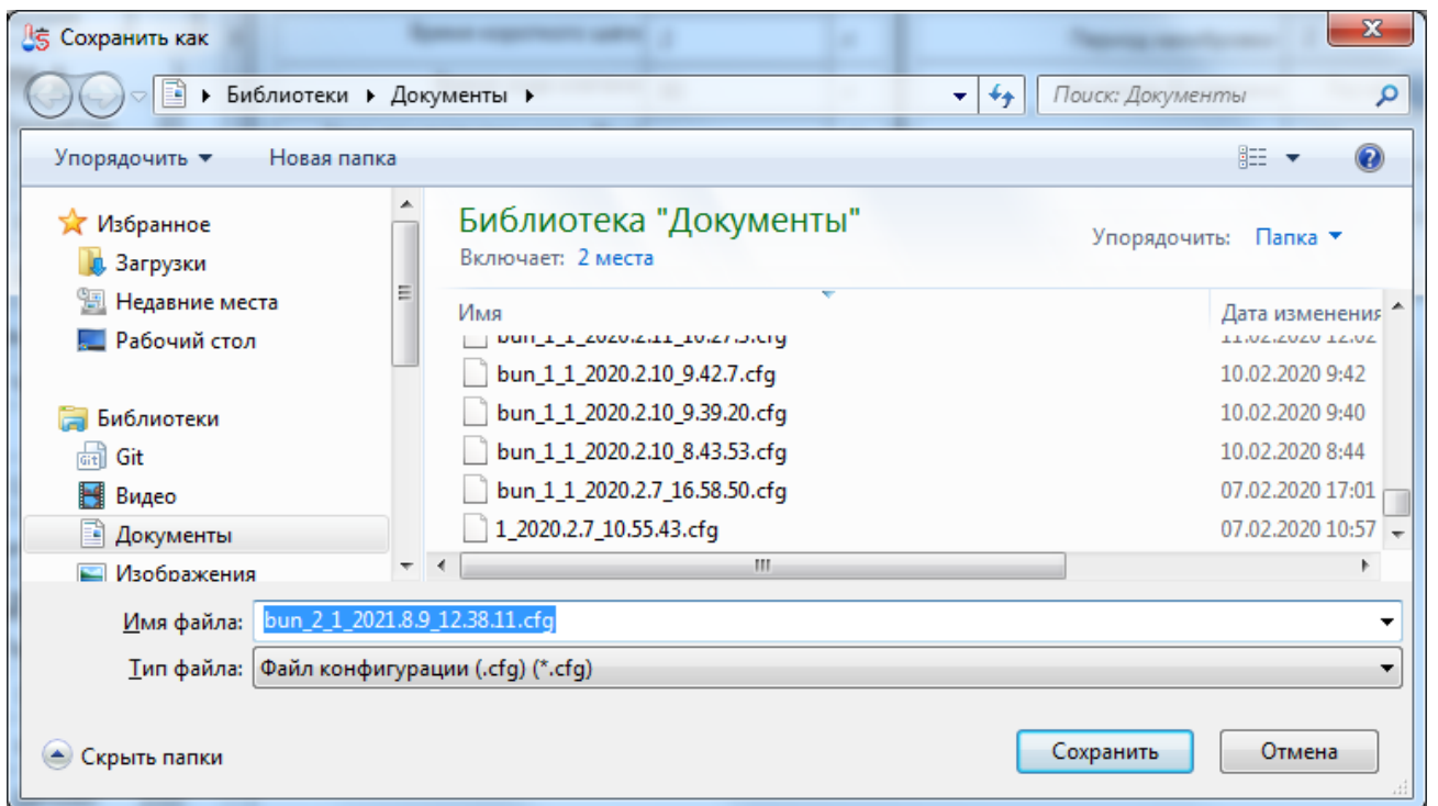
Рисунок 103 – окно сохранения
